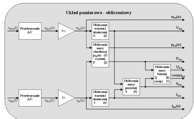
Rys. 3. Schemat blokowy układu pomiaru i obliczania parametrów instalacji elektrycznej
