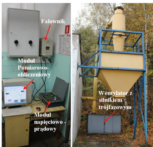
Rys. 4. Widok stanowiska pomiarowego Fig. 4. View of measuring stand
