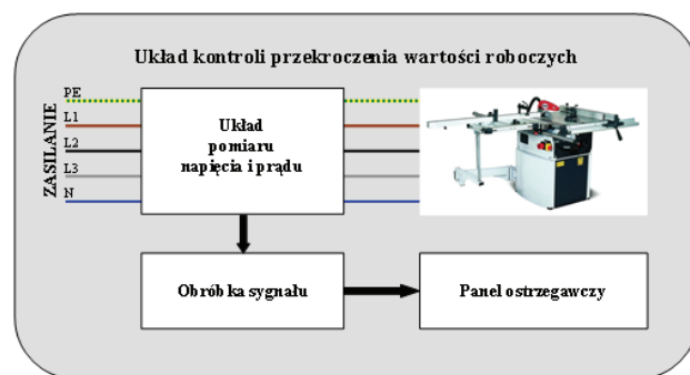
Rys. 11. Układ kontroli przekroczenia dopuszczalnych wartości technologicznych
