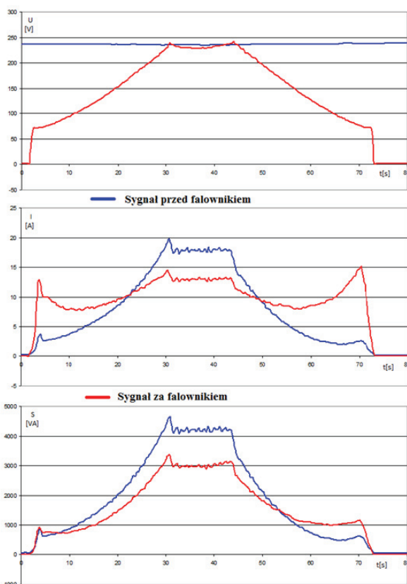
Rys. 7. Wykres wartości skutecznych podczas rozruchu silnika sterowanego falownikiem na wejściu oraz wyjściu falownika
